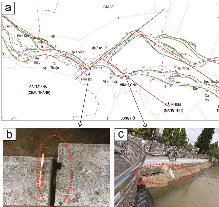
Hình 3. (a) Đoạn sông có hướng chảy thay đổi tại vị trí đi qua thành phố Vinh Long do hoạt động của đứt gãy Sông Tiên, (b, c) Bờ kè bị phá hủy do hoạt động của đứt gãy Sông Tiên.
