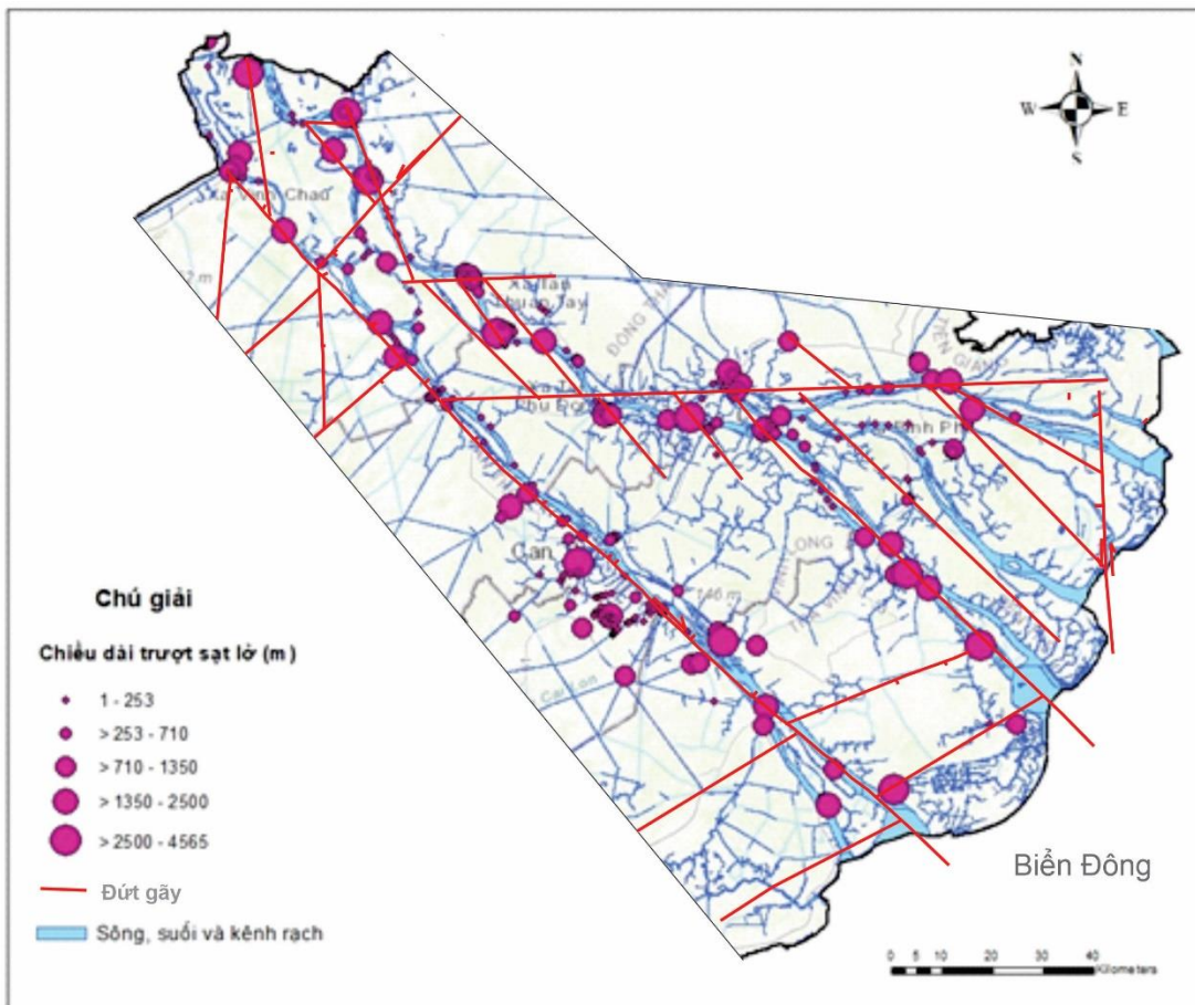
Hình 4. Sơ đồ tương quan giữa vị trí và quy mô các điểm xói lở trong vùng nghiên cứu với các đứt gãy hoạt động cho thấy hầu hết các điểm xói lở mạnh thường xảy ra ở vị trí giao nhau của các đứt gãy hoặc các vị trí đứt gãy hoạt động mạnh.
