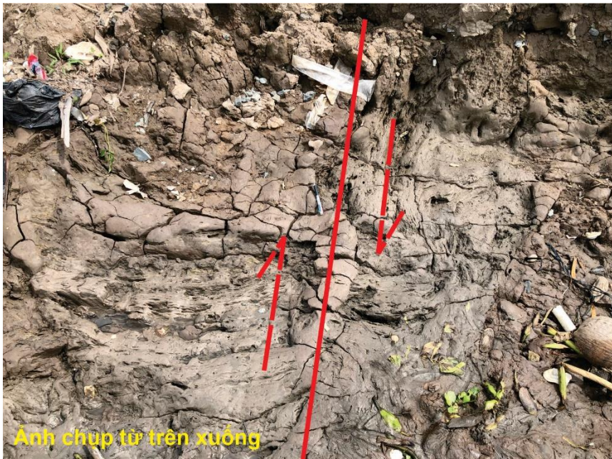
Hình 2. Hoạt động của đứt kiến tạo hoạt động dọc theo đứt gãy Sông Tiền làm dịch chuyển, biến dạng các thành tạo trầm tích trẻ tại vị trí khảo sát có tọa độ 10^{\circ}19'28.0'' - 106^{\circ}14'42.0'' .
